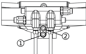
(图5) 车头螺丝锁固顺序
