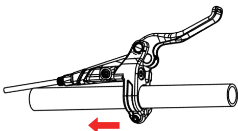
(图5) 调整上泵位置与角度
