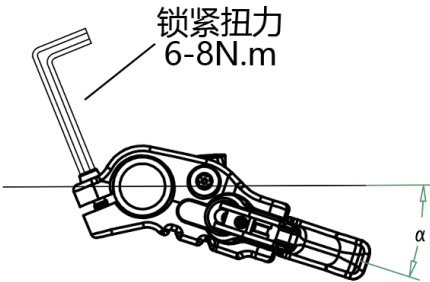
(图6) 束仔螺丝锁紧扭力
